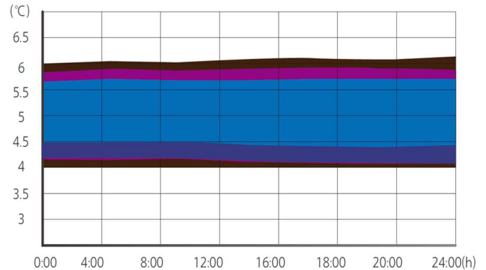
温度均一性
