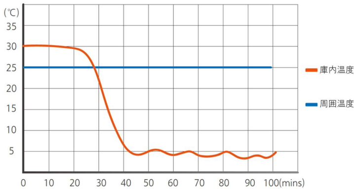
温度カーブ
