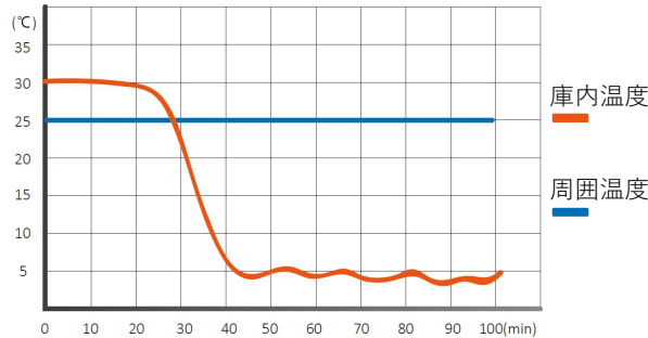
冷却時温度カーブ
