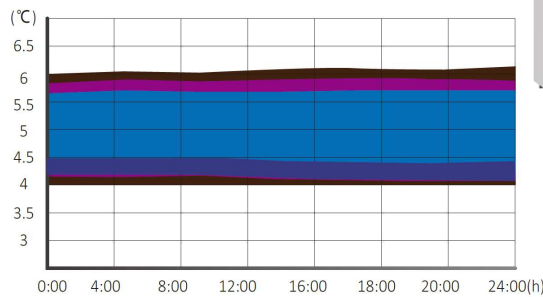
庫内温度均一性
